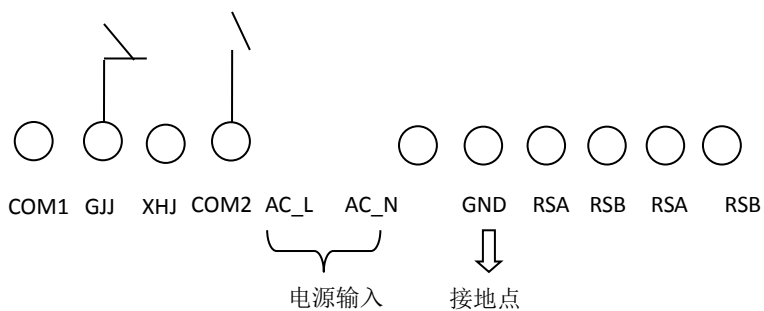
图 6 端子结构示意图
