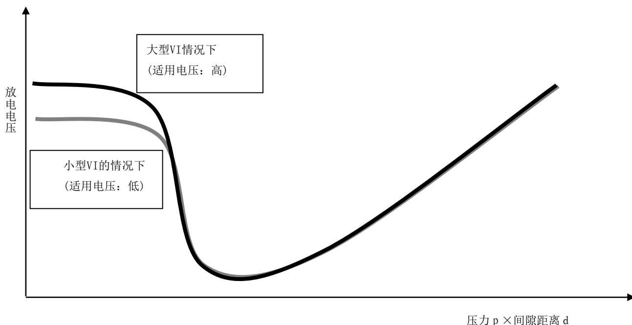
图 2 帕邢曲线
